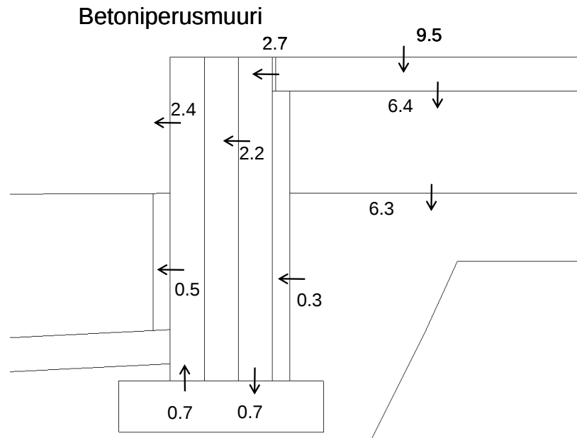
Kuva 14. Lämpövirrat (W/m) jatkuvuustilanteessa rakenteiden rajapinnoissa kun ulkolämpötila on 0 °C ja lattian pintalämpötila 20 °C. Perusmuuri on betonia.
