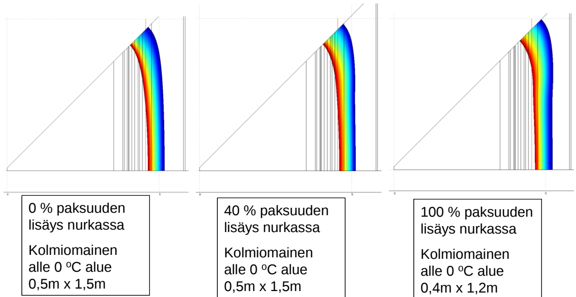
Kuva 20. Lämpötila-alue -1^{\circ}\text{C} \dots 0^{\circ}\text{C} 200 mm anturan alapuolella nurkan läheisyydessä 24. maaliskuuta Jyväskylässä ylhäältä katsottuna. Rakenne ja eristykset ovat muuten samat kuin kuvan 9 2-ulotteisissa laskelmissa mutta nurkassa eristyspaksuutta on lisätty 0 %, 40 % tai 100 %.
