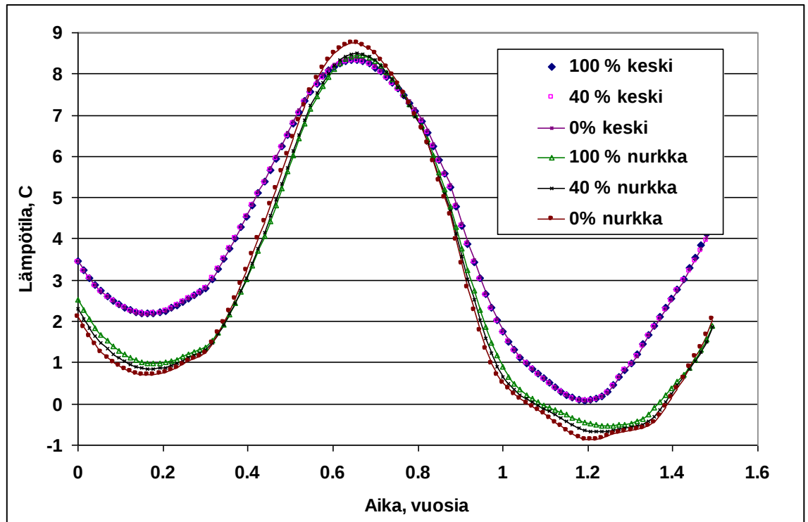
Kuva 21. Tarkastelupisteen lämpötilat seinän keskellä ja nurkassa. Rakenne ja eristykset ovat muuten samat kuin kuvan 9 kaksikulotteisissa laskelmissa mutta nurkassa eristyspaksuutta on lisätty 0 %, 40 % tai 100 %.
