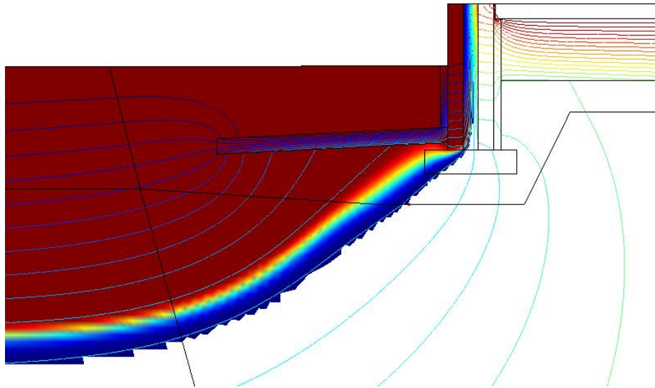
Kuva 9. Roudan eteneminen kylmänä talvena maaliskuun 12. päivänä Jyväskylässä. Väritetyn alueen lämpötila on nolla-asteen alapuolella. Kuvassa on myös isotermit yhden asteen välein. Lattiaeristeen paksuus on 400 mm, routaeristeen leveys 1,5 m ja paksuus 100 mm.
