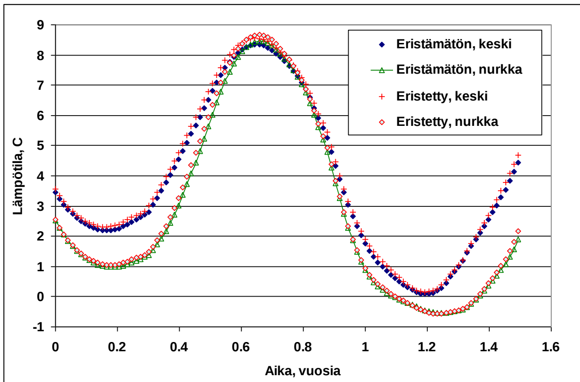
Kuva 23. Tarkastelupisteen lämpötilat seinän keskellä ja nurkassa kun nurkassa on kaksinkertainen eristyspaksuus seinä-alueeseen verrattuna. Perusmuuri on joko kuvan 2 mukainen, tai ulkopuolelta ylös asti 50 mm eristeellä eristetty. Routaeristeen paksuudet ovat vastaavasti 100 mm tai 65 mm ja leveys on 1,5 m.
