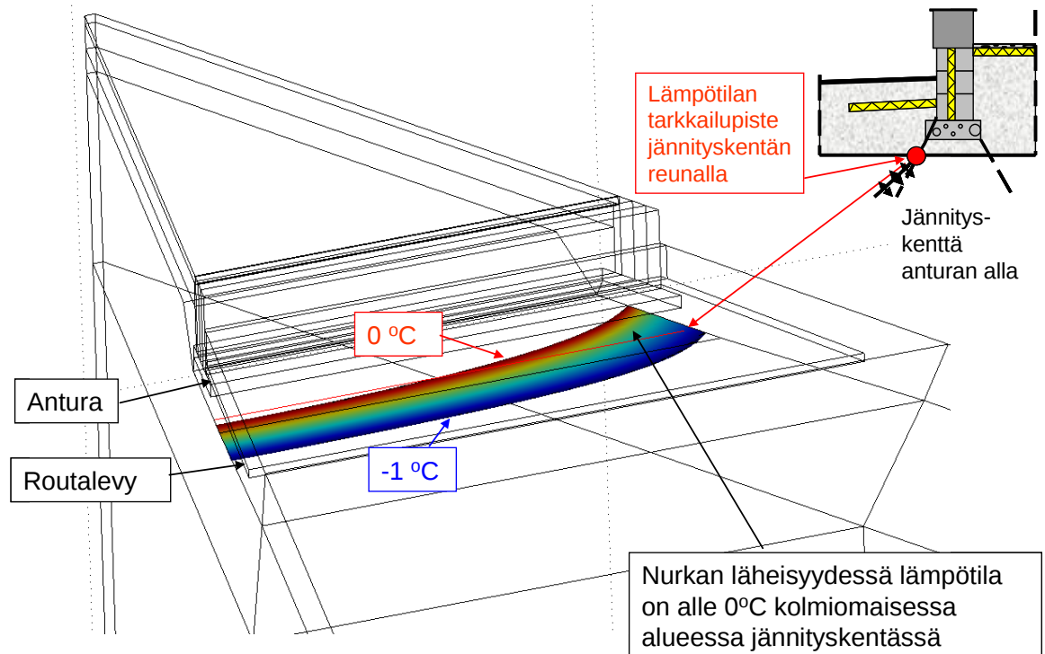
Kuva 19. Lämpötila-alue -1^{\circ}\text{C} ... 0^{\circ}\text{C} 200 mm anturan alapuolella nurkan läheisyydessä 24. maaliskuuta Jyväskylässä. Rakenne ja eristykset ovat samat kuin kuvan 9 kaksiulotteisissa laskelmissa. Laskenta-alue selviää kuvasta 18.
